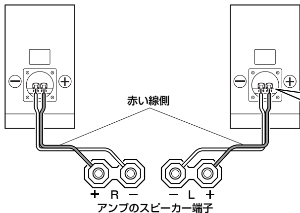
右側(Rチャンネル)の スピーカー
